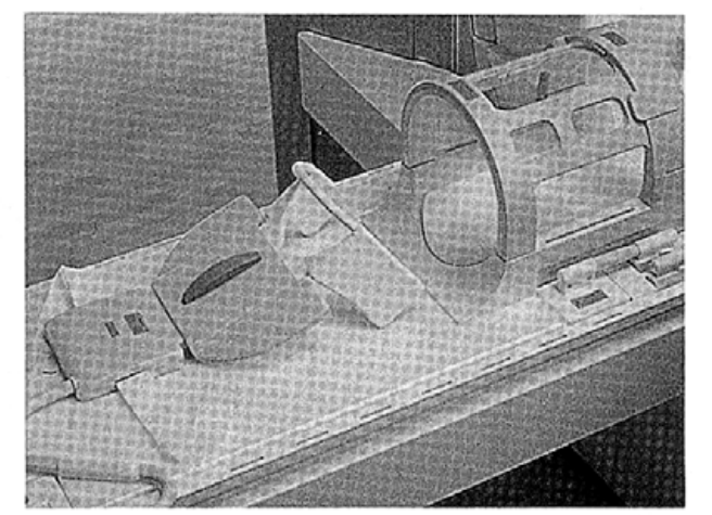
新しく導入された高磁場MRI「ハーモニー」
